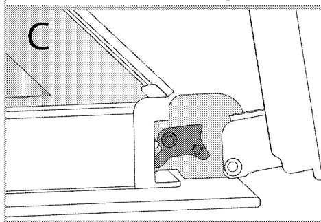
Bloqueo de la bisagra - posición abierta 3. Lleve la puerta del horno a una posición semiabierta.
