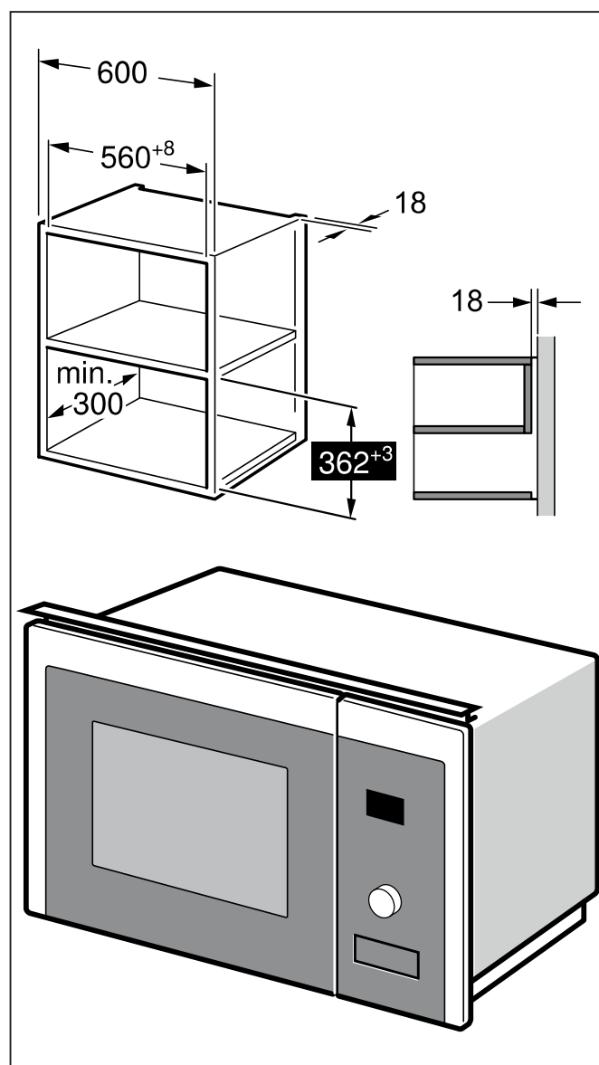
Installation dans un meuble mural suspendu
